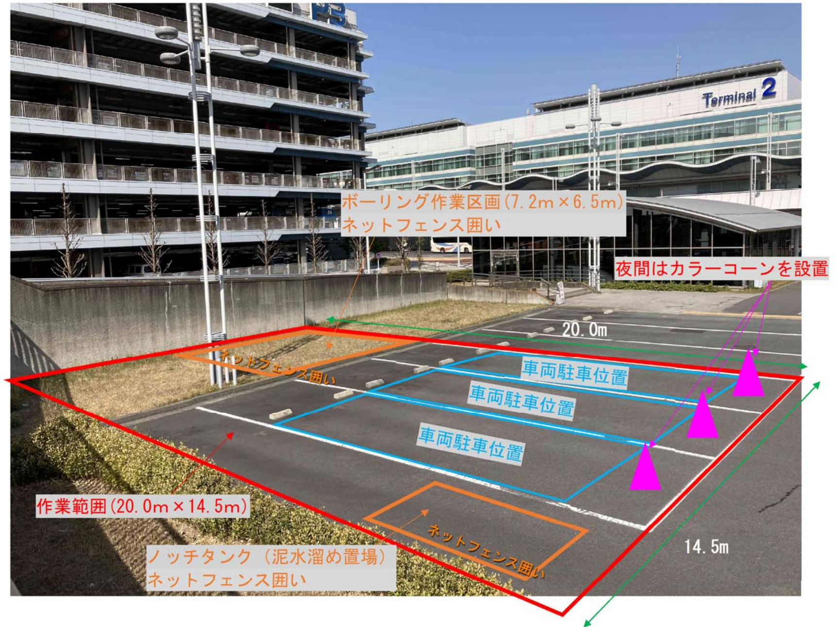
No. 3ボーリング調査 作業範囲図
